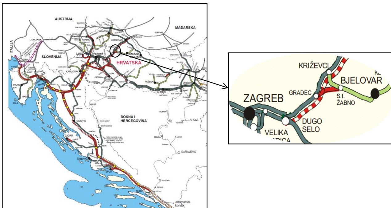
Slika 1 – Prostorni i situacijski prikaz dionice Gradec - Sveti Ivan Žabno
