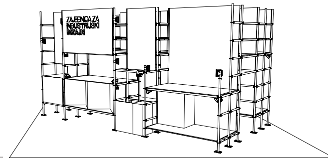
PERSPEKTIVA STRANA 1
