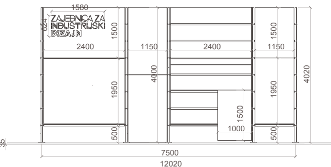
BOKOCRT
