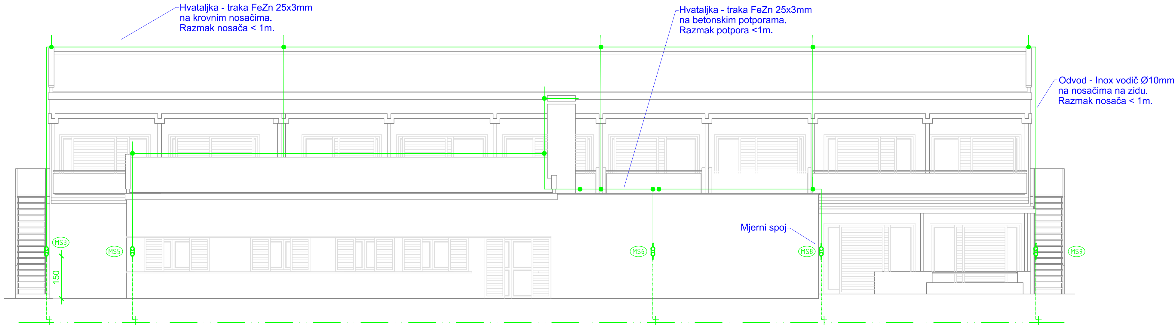
SJEVEROZAPADNO PROČELJE
