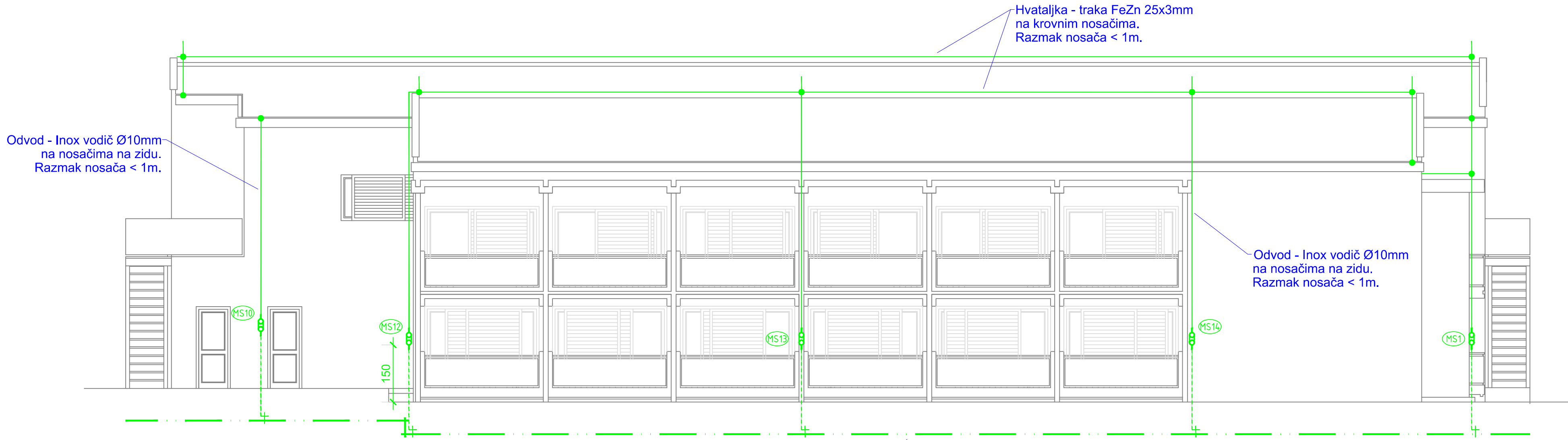
JUGOISTOČNO PROČELJE
