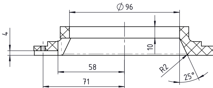
Presjek A-A
