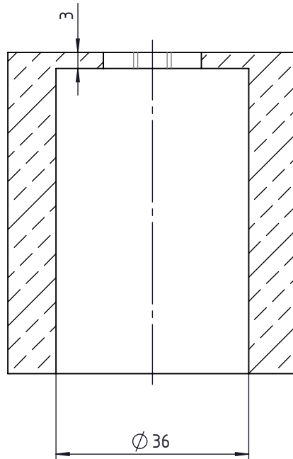
Presjek A-A
