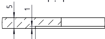
Detalj B 1 : 1
