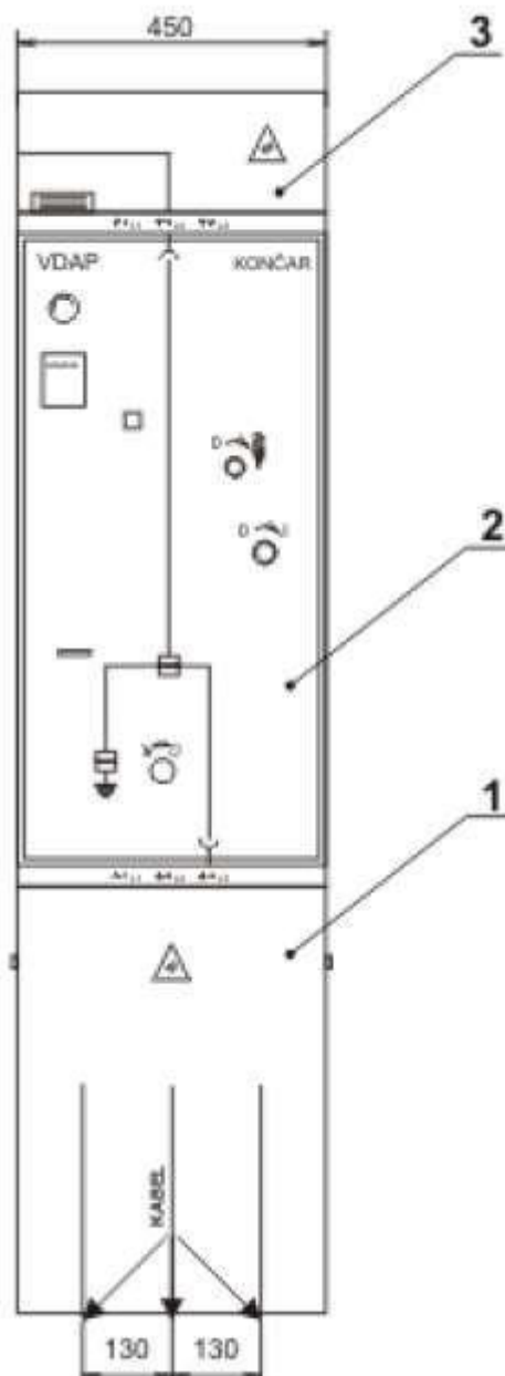
Slika – Mjerna skica sklopnog modula serije VDAP
