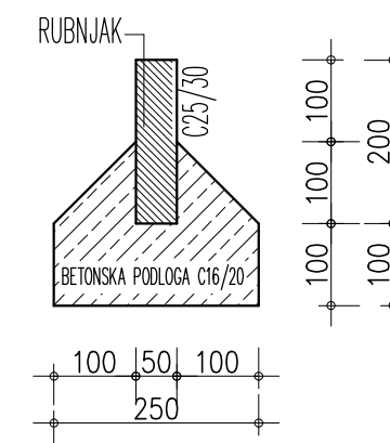
BETONSKI RUBNJAK 5/20 M 1:10
